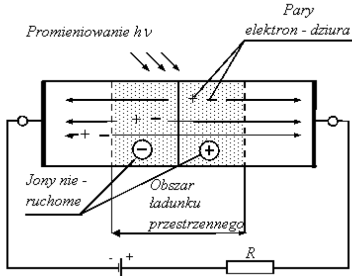
Rys. 1.1. Zasada działania fotodiody
