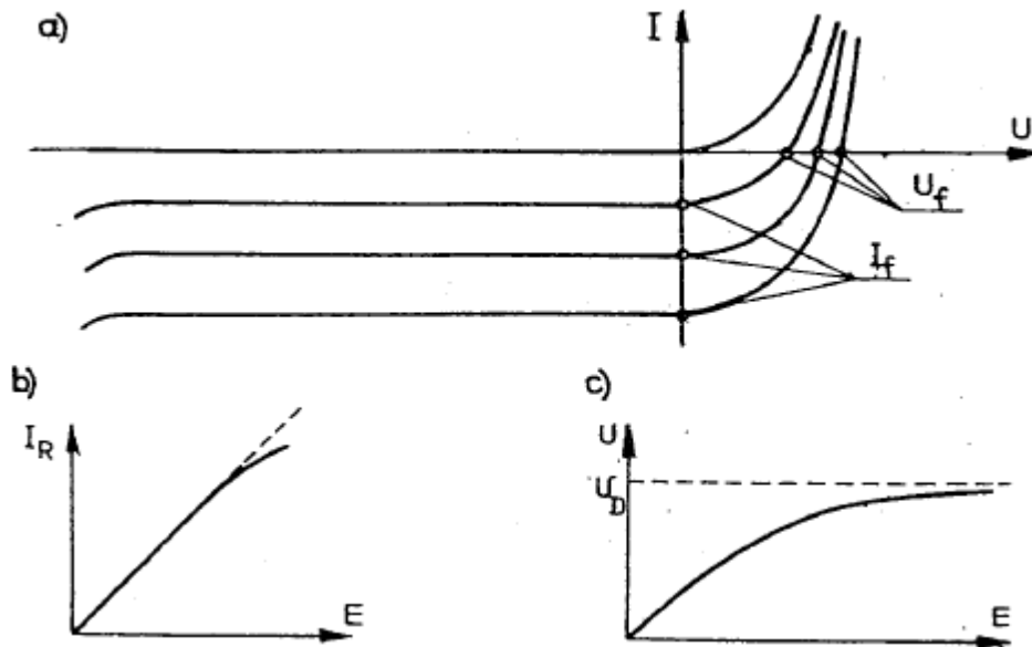
Rys. 1.2. Charakterystyki statyczne fotodiody: a) prądowo napięciowa, b) zależności prądu wstecznego od natężenia oświetlenia, c) zależności napięcia fotoelektrycznego od natężenia oświetlenia
