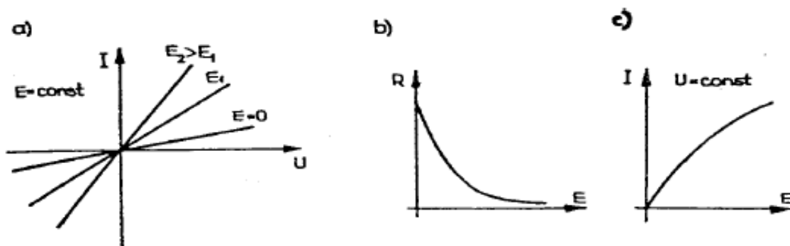
Rys. 2.2. Charakterystyki fotorezystora: a) prądowo – napięciowa przy stałym natężeniu, b) rezystancji od natężenia oświetlenia, c) świetlna
